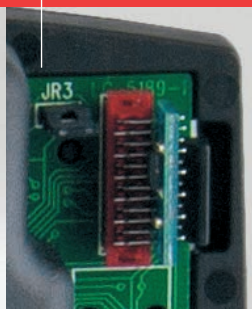
Memoria extraíble para guardar los parámetros
